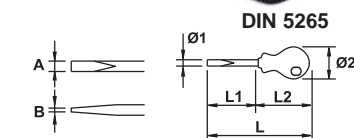
DIN 5265
